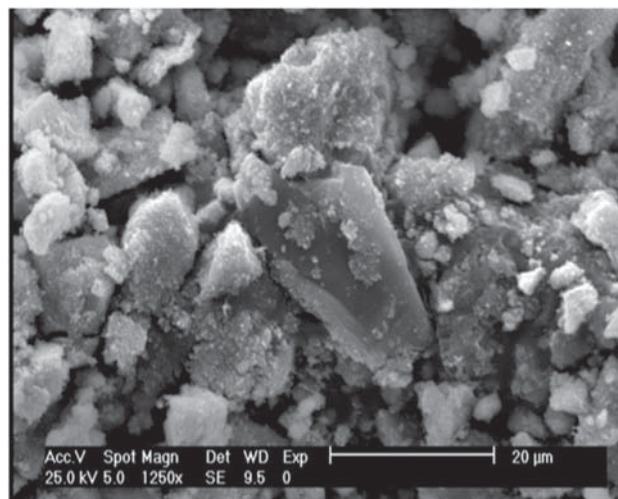
شکل ۳- نانوکاتالیست Fe_2O_3
